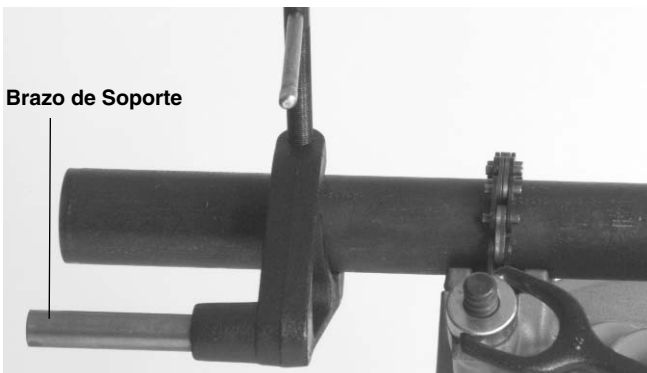
Figure 4 – Empleo del Brazo de Soporte No. 691 cuando se rosca un tubo de 3/4 pulgada o mayor
